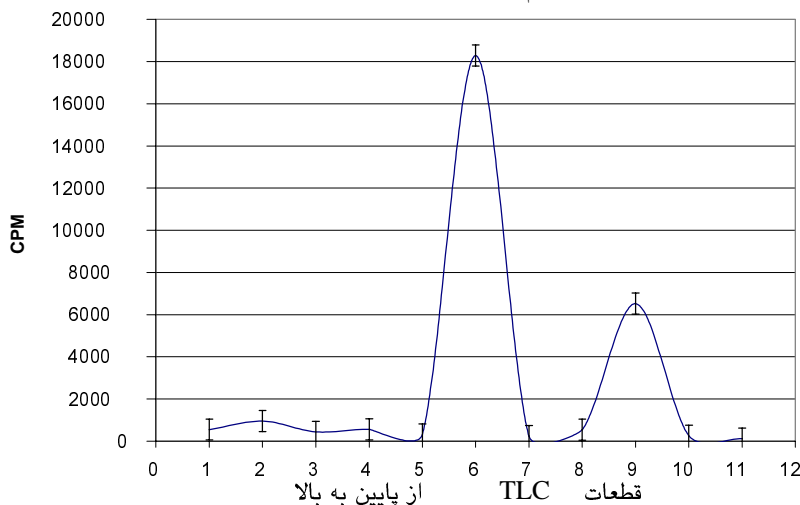
نمودار-۱: رادیوکروماتوگرام [^{111}\text{In}] - ایندیوم بلئومایسین در سیستم فاز متحرک متانول-آمونیم استات ۹ و ۱ ( R_{fA2}=0.27 & R_{fB2}=0.70 )
