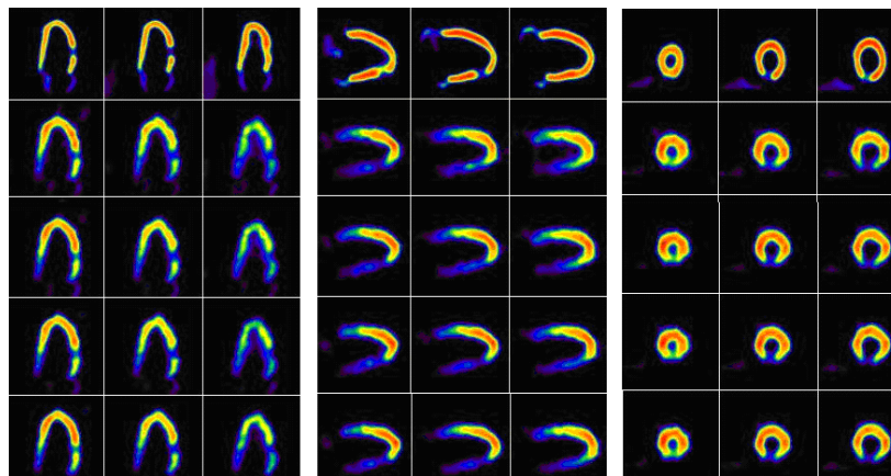
شکل ۲- به ترتیب از بالا به پایین: تصویر فانتوم اکتیوته NCAT (تصویر مرجع)، تصویر در پنجره متداول (۶۷-/۲۰ keV) و پنجره های مورد بررسی به ترتیب (۷۳-/۳۰ keV) و (۷۵-/۳۰ keV) و (۷۷-/۳۰ keV). از چپ به راست به ترتیب مقاطع sagittal ، axial و coronal
