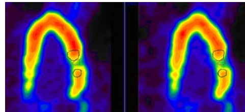
شکل ۳ - طریقه رسم ROI جهت محاسبه کنتراست دیواره به ضایه در قلب
