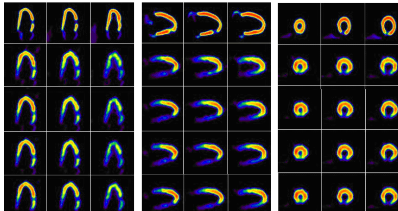
شکل ۲- به ترتیب از بالا به پایین: تصویر فانتوم اکتیو NCAT (تصویر مرجع)، تصویر در پنجره متداول (۶۷-۲۰ keV) و پنجره های مورد بررسی به ترتیب (۷۳-۳۰ keV) و (۷۵-۳۰ keV) و (۷۷-۳۰ keV). از چپ به راست به ترتیب مقاطع sagittal، coronal و axial
