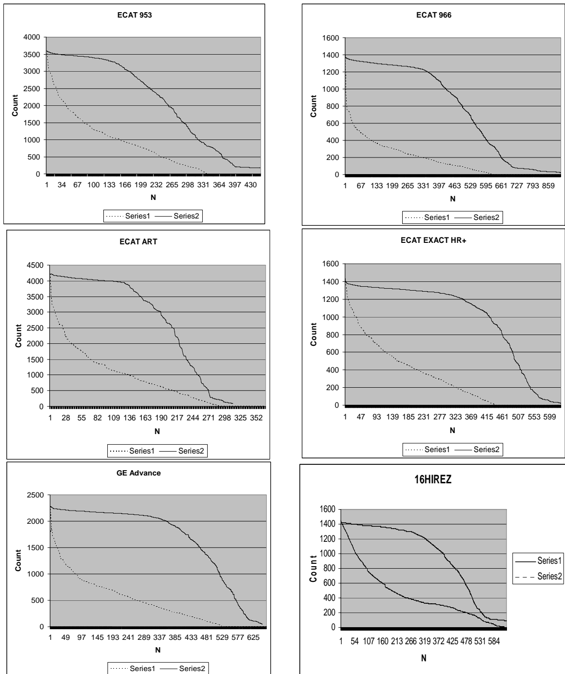
شکل ۳- نمودار مربوط به کانت کلیه پیکسل های قرار گرفته در درون ROI پس از نرمالایز شدن کانت تصاویر بازسازی شده (نمودارهای خط چین) بر حسب مقادیر مربوط به تصاویر مرجع (نمودارهای خط پیوسته).
